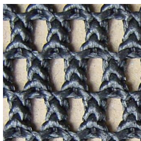
ラッセル織り黒着色 繊維量 700g+樹脂(1㎡当)
